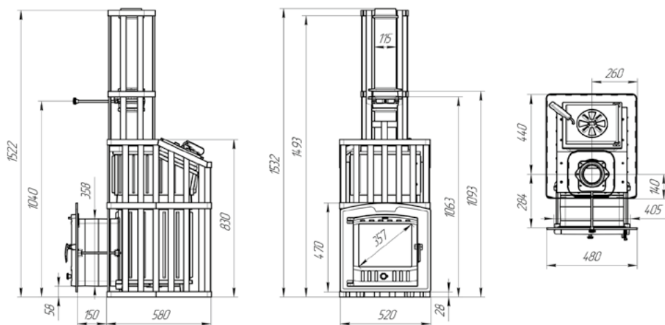
Рис. 2.1 Размеры печи Гроза 18П2 (комплектация Ураган)
