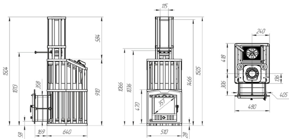
Рис. 2.2 Размеры печи Гроза 24П2 (комплектация Ураган)
